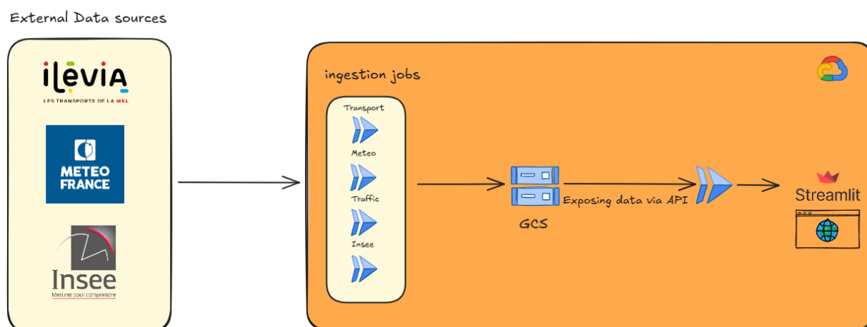
Figure 2 : Schéma du Projet Open Data
