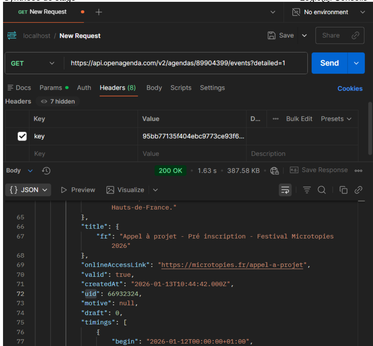
Figure 3: Capture d'écran de Postman lors d'une réponse à une requête HTTP
