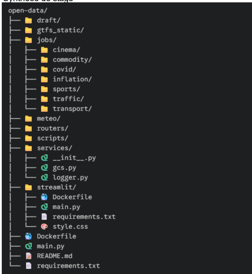
Structure du Git et du projet Open Data
